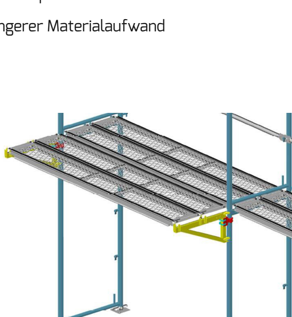
Einsatz Variable Konsole SL 2-bohlig
