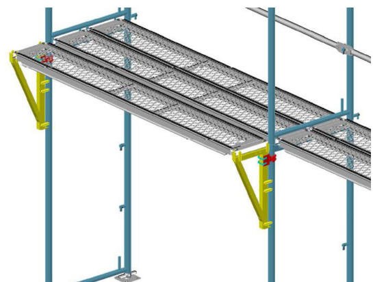
Einsatz Variable Konsole SL 1-bohlig
